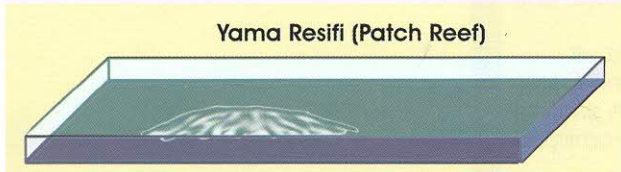
Şekil 10. Sınırlı alanda gelişen karbonat yığılımları yama resifi olarak bilinir.
