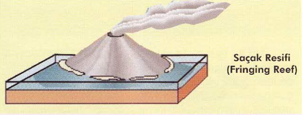
Şekil 12. Kara ile resif gelişim arasında bir lagün yok, resif doğrudan karaya bağlanıyor ise saçak resifi adını alır.
